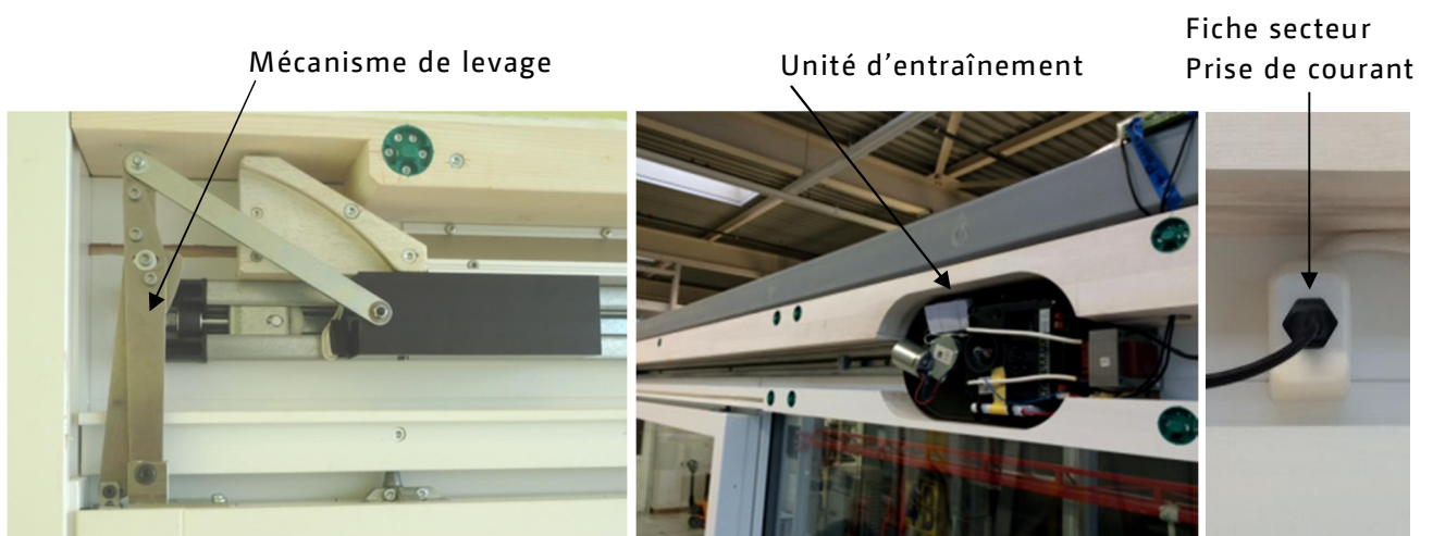
Image 3 : Élargissement supérieur du cadre Vantail fermé et verrouillé
