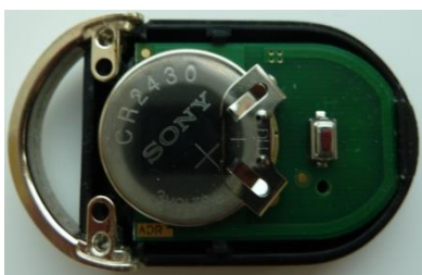
Image 10 : Pile CR 2430, 3 V
