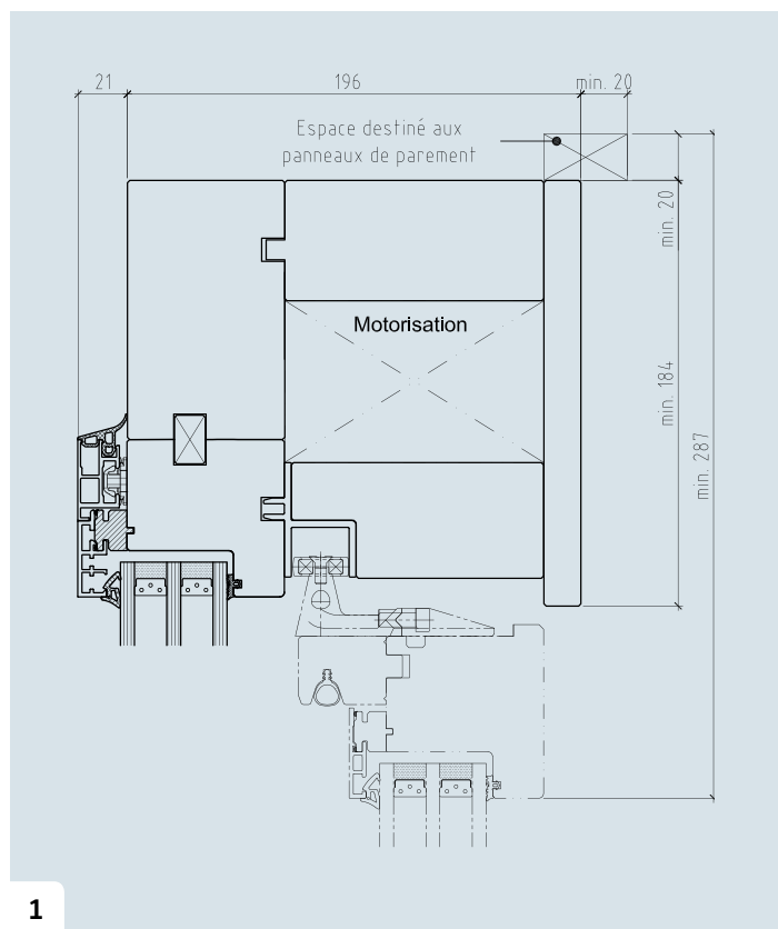
Partie fixe, coupe supérieure, type GL
