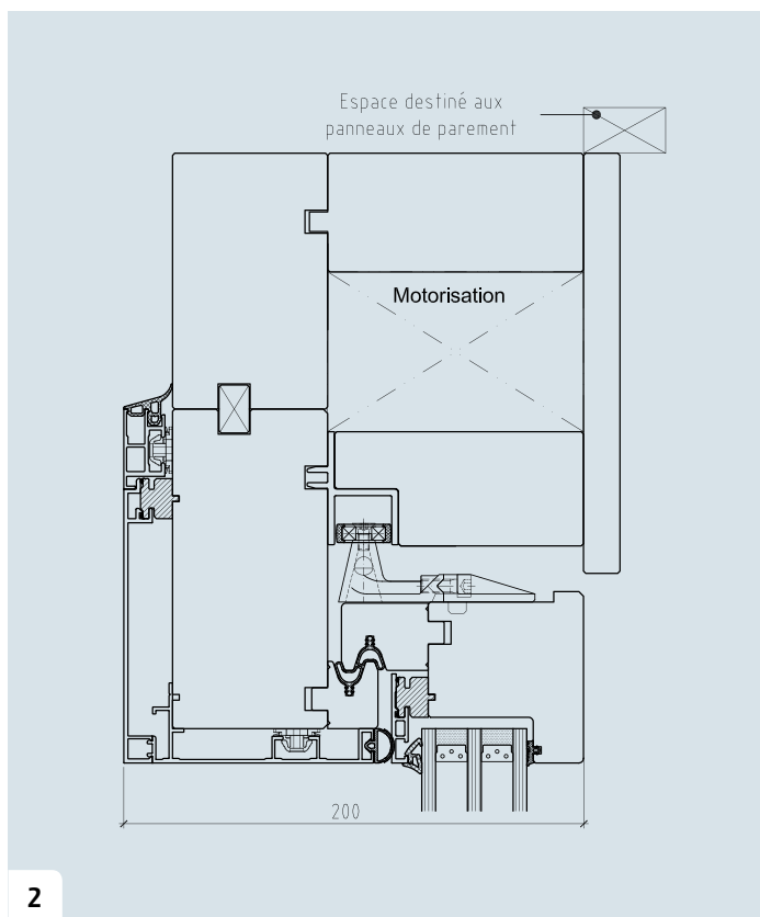
Passage, coupe supérieure
