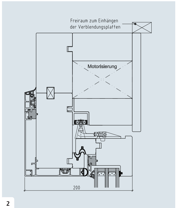
2 Durchgang, Schnitt oben
