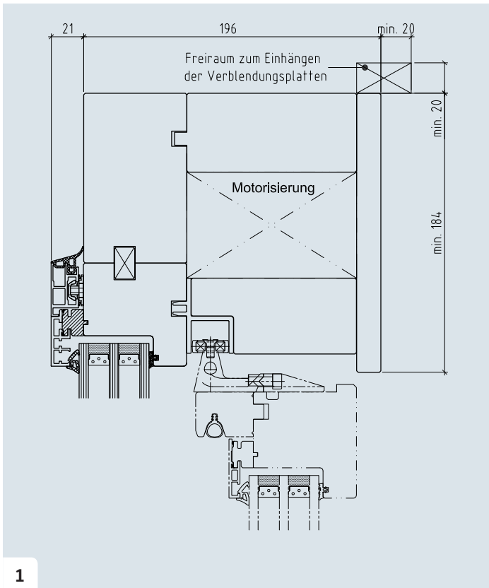
1 Festteil, Schnitt oben, Typ GL
